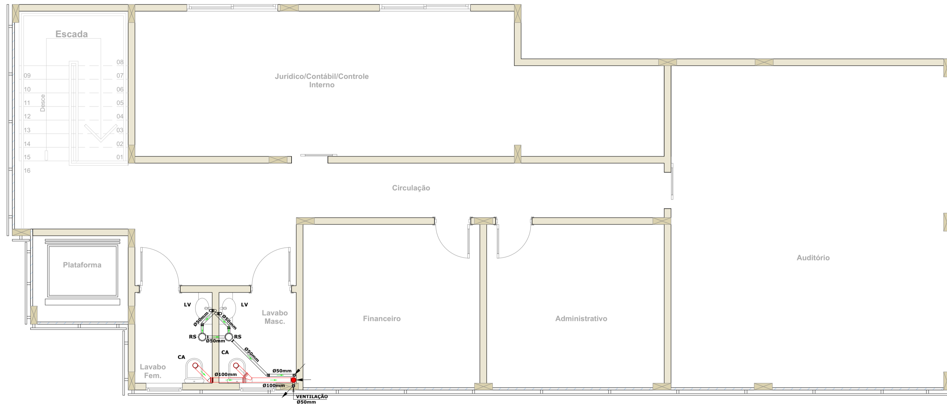
PLANTA BAIXA SEGUNDO PAV. PROJETO SANITÁRIO ESCALA 1/50
