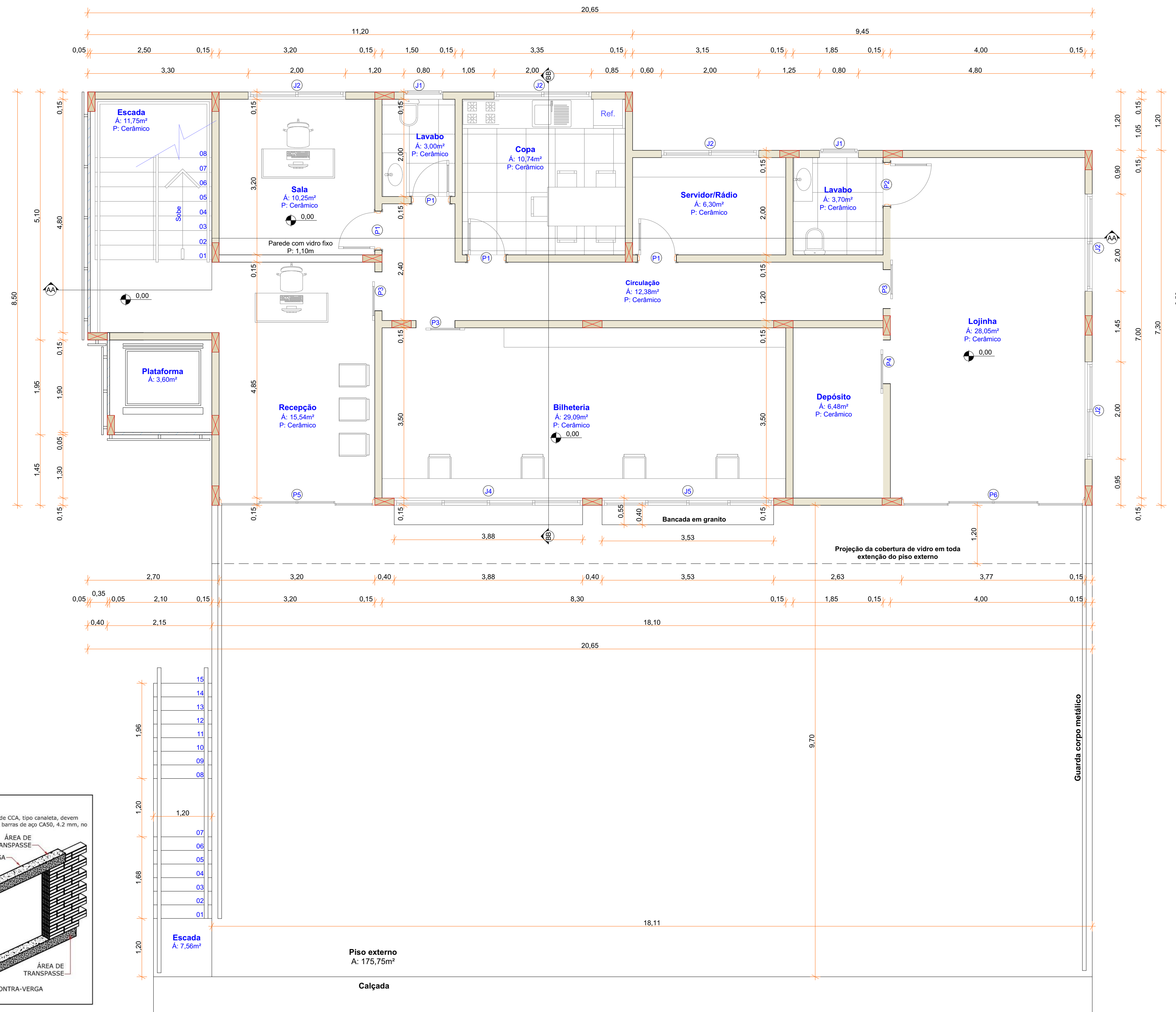
PLANTA BAIXA PAV. TÉRREO ESCALA 1/50
