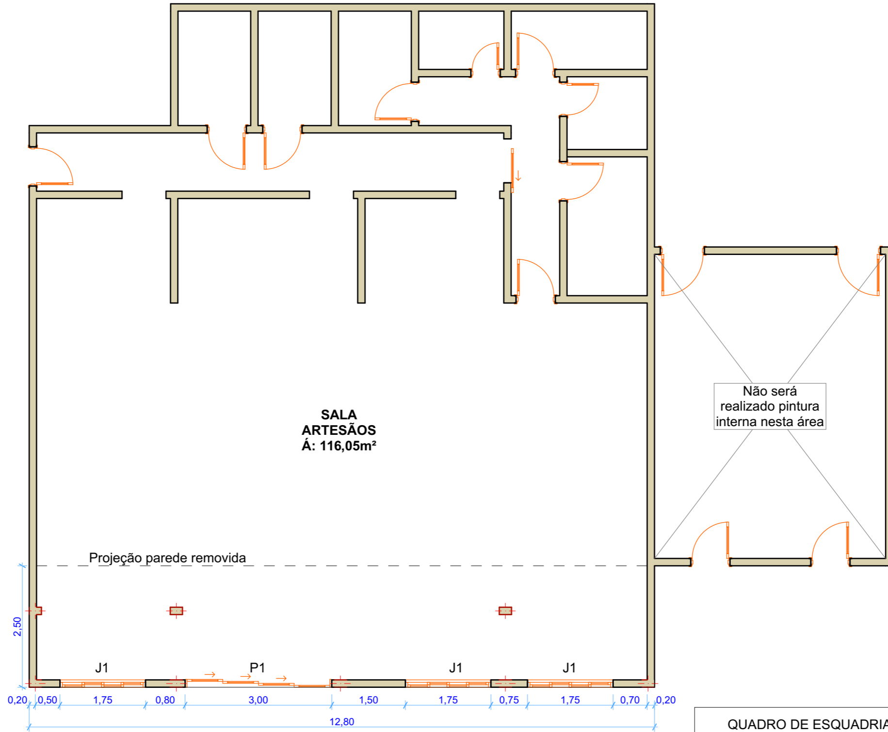
PLANTA BAIXA FINAL ESCALA: 1/75
