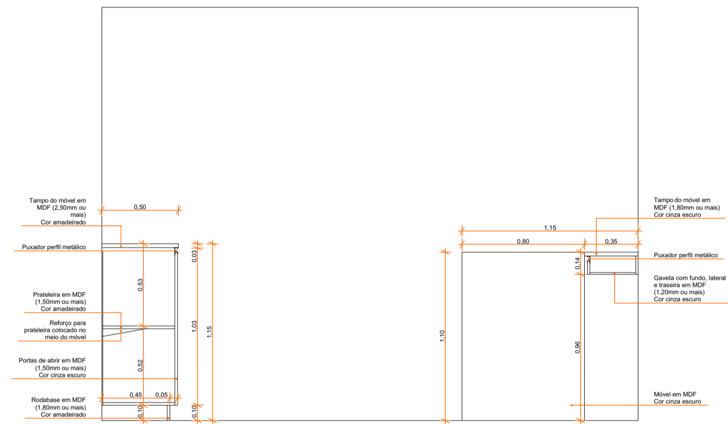
BILHETERIA VISTA 02 ESCALA: 1/25
