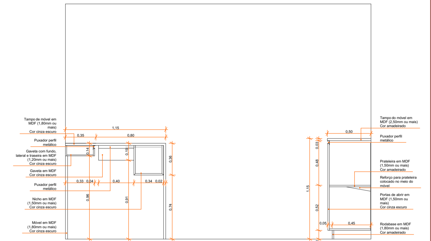
BILHETERIA VISTA 04 ESCALA: 1/25
