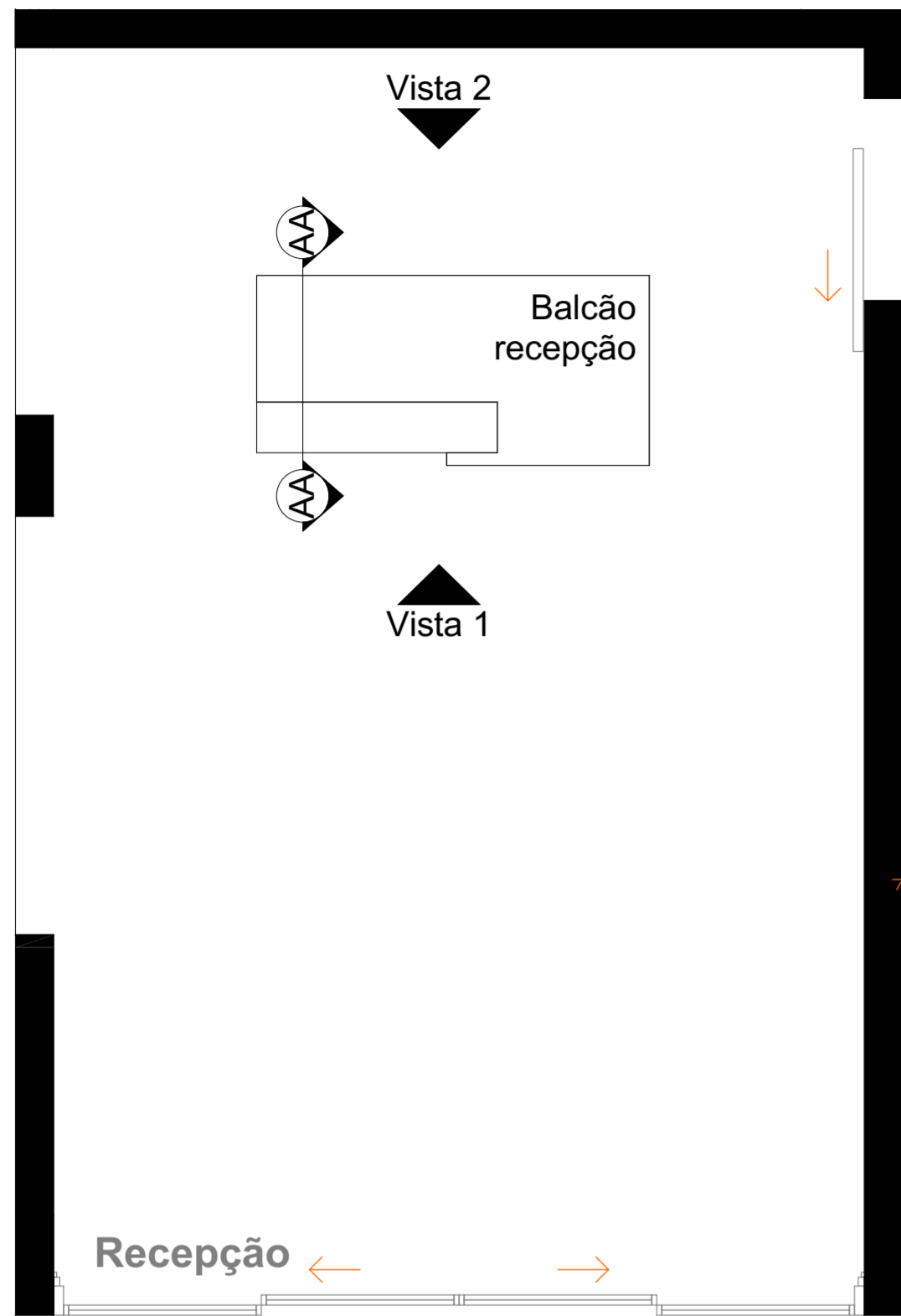
PLANTA LAYOUT ESCALA: 1/25
