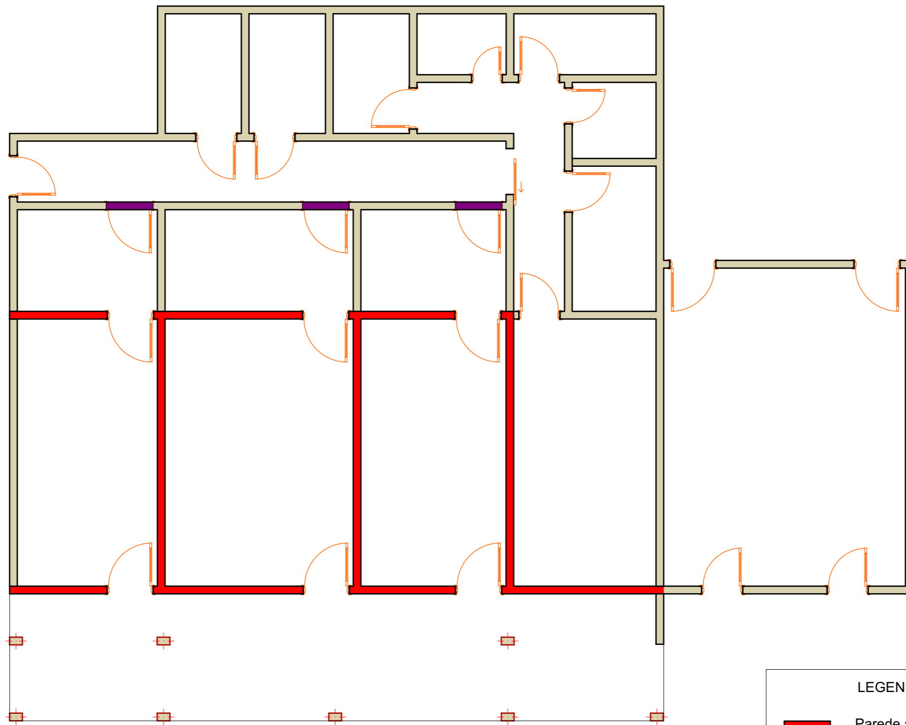
PLANTA BAIXA DEMOLIÇÕES ESCALA: 1/75
