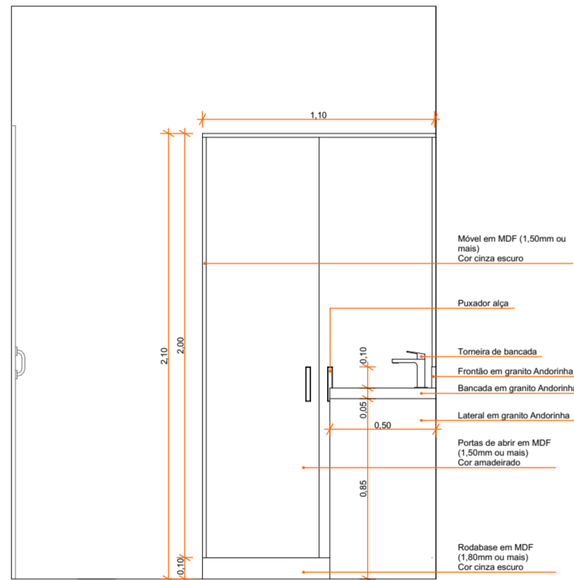
LAVABO VISTA 02 ESCALA: 1/25
