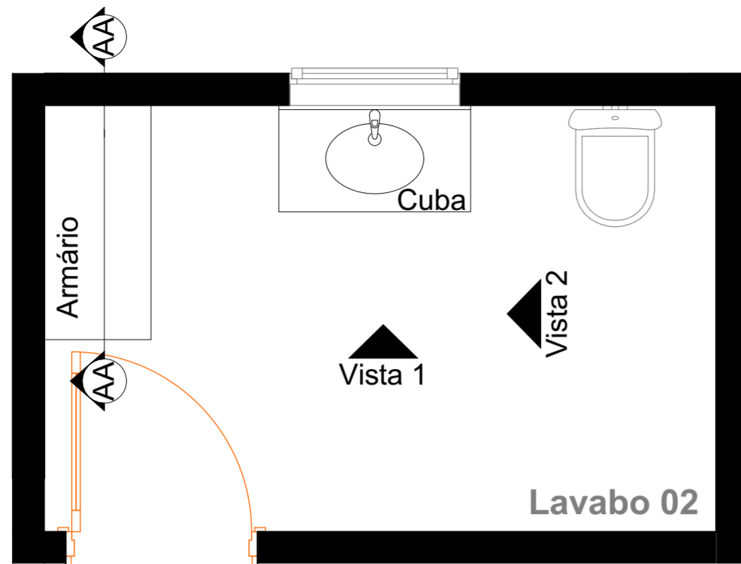
PLANTA LAYOUT ESCALA: 1/25
