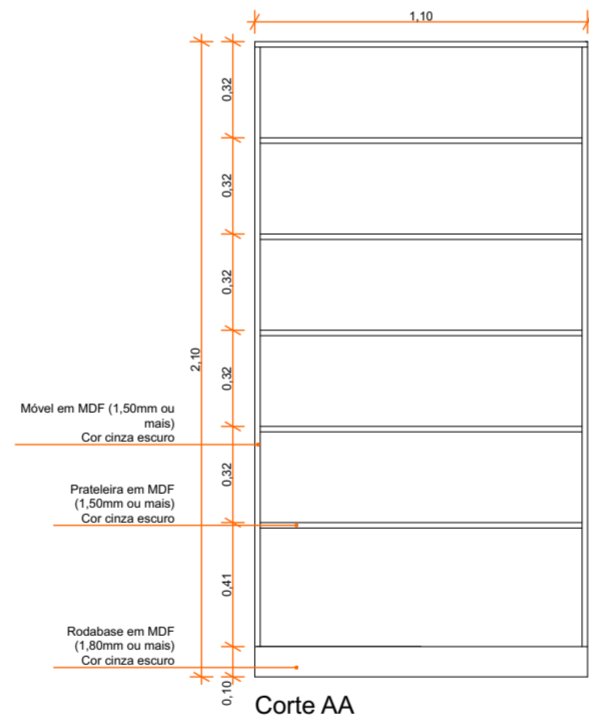
Corte AA
