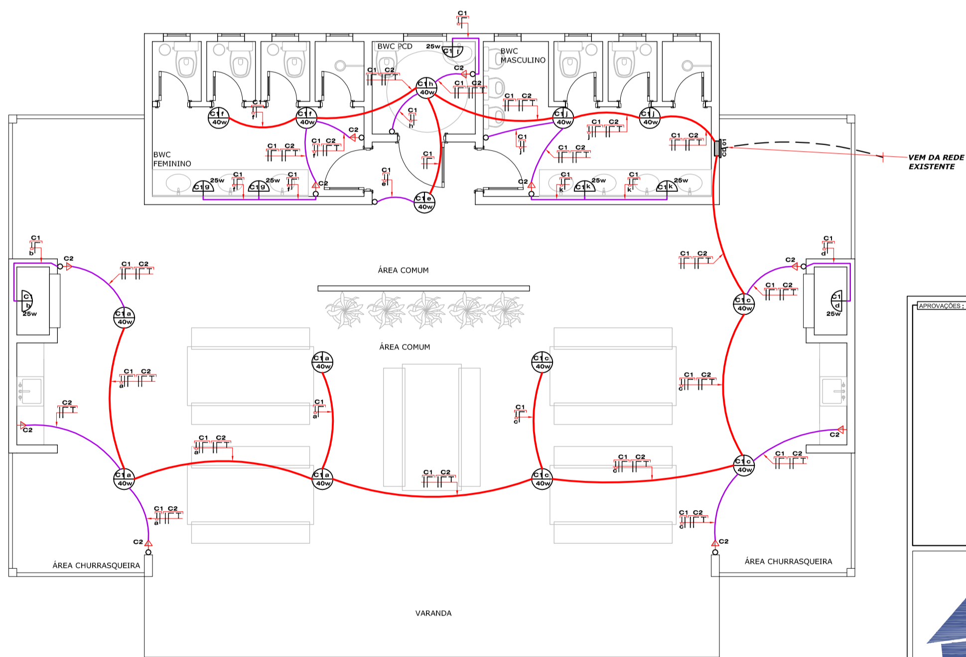
PLANTA BAIXA PROJETO ELÉTRICO ESCALA = 1 : 50
