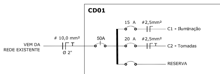
DIAGRAMA UNIFILAR SEM ESCALA
