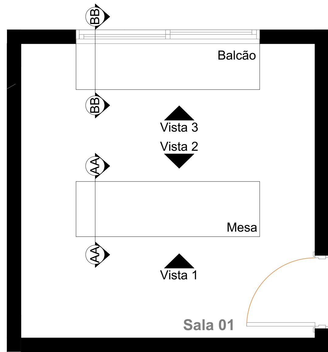
PLANTA LAYOUT ESCALA: 1/25
